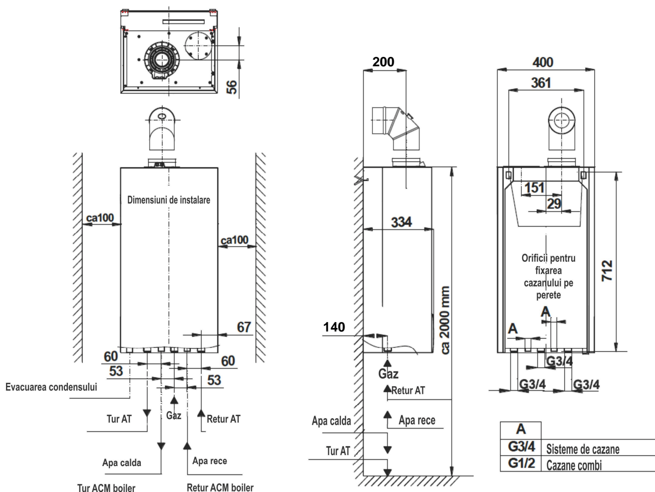
Img. 3.3.1. Dimensiuni de instalare pentru cazanele ECOCONDENS SILVER PLUS
