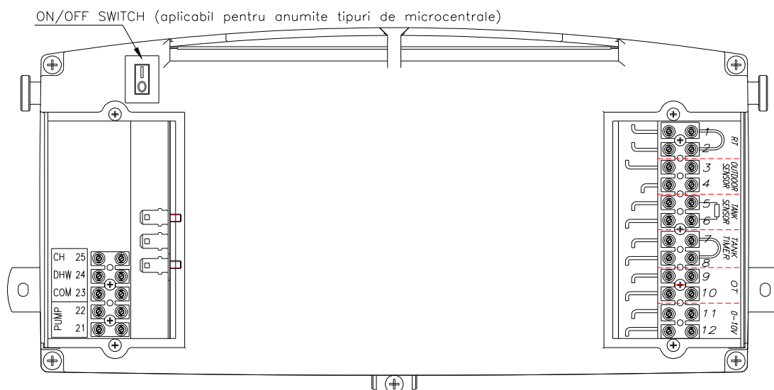
Fig.3.9.1 Conexiunii electrice in cazul centralelor combi
