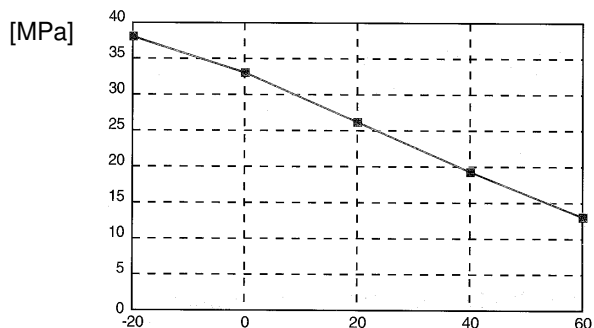
Variatia cu temperatura (T - °C) a solicitării la traciune (MPa).
