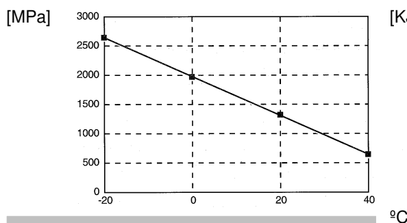
Variatia cu temperatura (T - °C) a modului de elasticitate la traciune (E - MPa).
