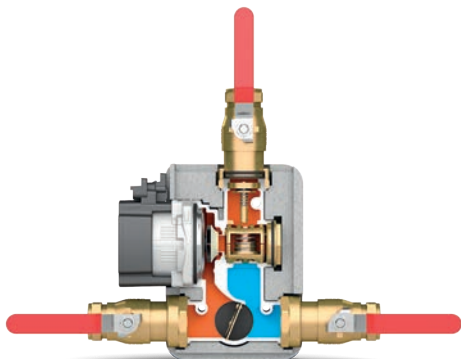
Takaisku- ja vapaavirtausventtiili on vakiovaruste. Backventil/själv-cirkulationsventil är standard. The return flow preventer/self circulation valve is standard. Der Rückflussverhinderer/das Selbstzirkulationsventil ist Standard.
