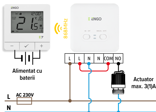
c) Diagrama de conexiune pentru actuator
