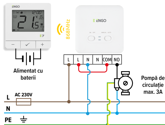
b) Diagrama de conexiune pentru pompe de circulație
