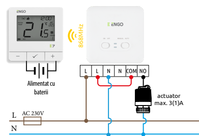
c) Diagrama de conexiune pentru actuator
