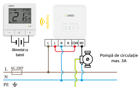
b) Diagrama de conexiune pentru pompe de circulație
